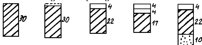
Rys. 4. Przykładowe wybrane konstrukcje nawierzchni utwardzonego pobocza z kruszywem łamanym niezwiązanym
